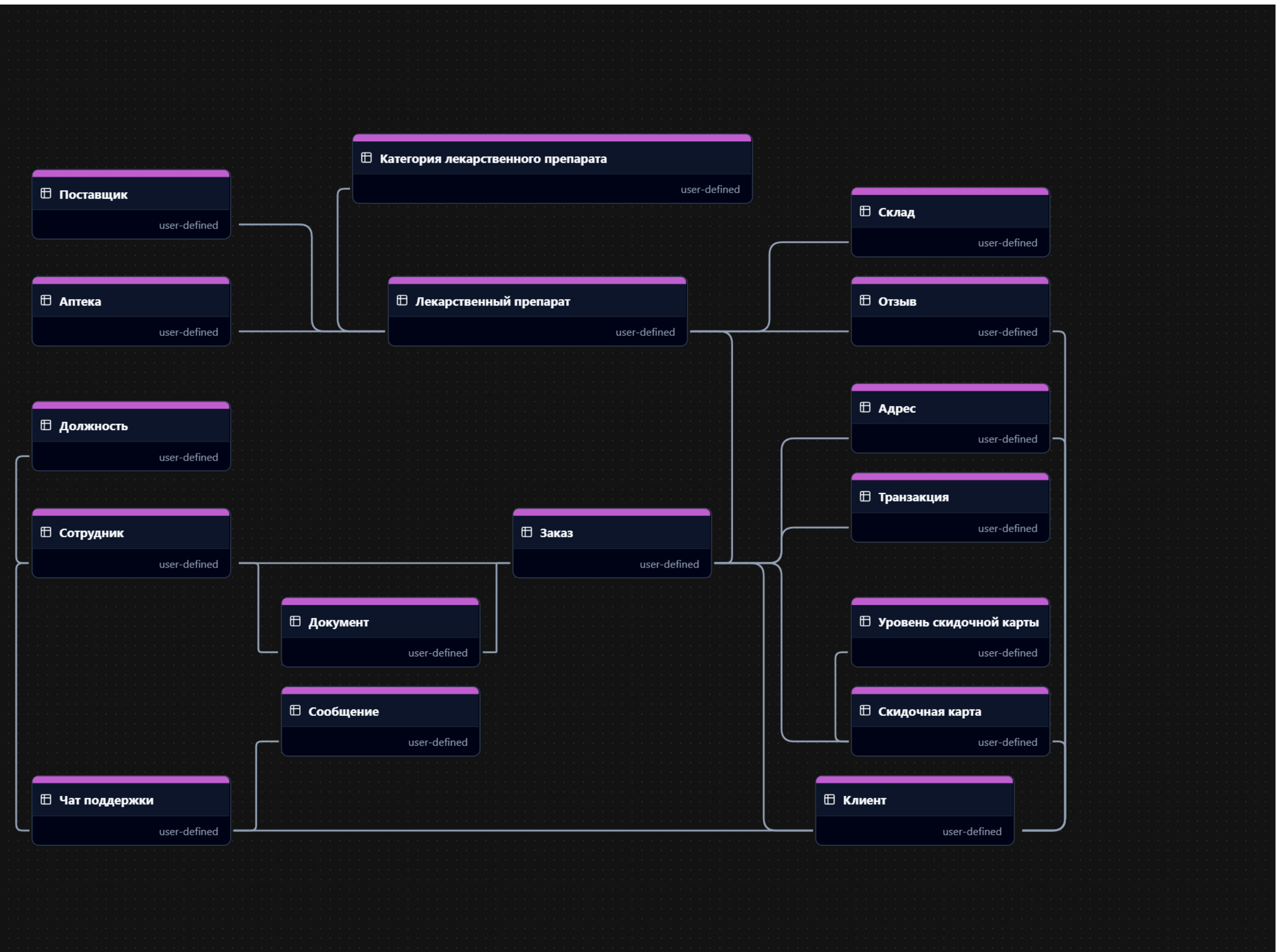
Рисунок 1 — Концептуальная схема данных
